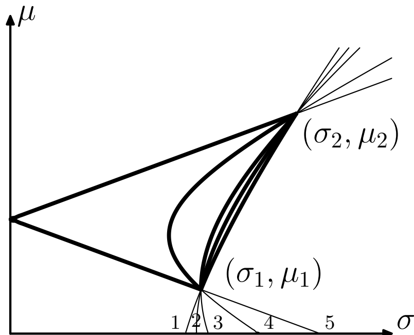
Joonis 3.3: Portfellide oodatav tulusused ja standardhälbed sõltuvalt \rho_{12} väärtusest. Jooned 1 ja 2: \rho_{12} > \sigma_1/\sigma_2 , jooned 4 ja 5: \rho_{12} < \sigma_1/\sigma_2 , joon 3: \rho_{12} = \sigma_1/\sigma_2 .
