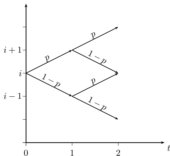
[Joonis: osakese liikumine ajas]
